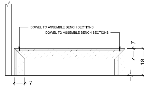
FOYER BENCH SCALE: 1/2" = 1'0"
