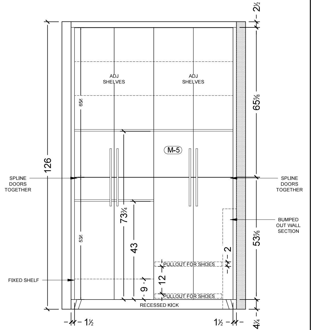
2 GUEST ENSUITE CLOSET ELEV SCALE: 1/2" = 1'0"
