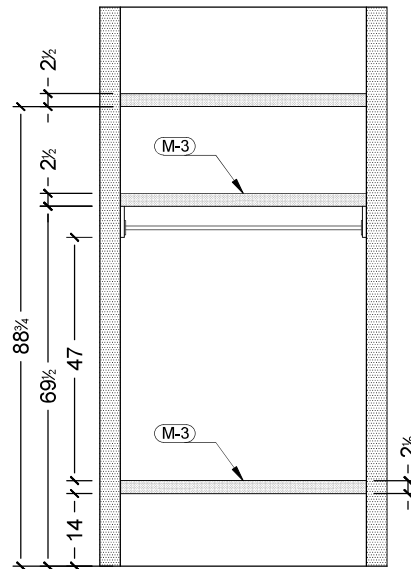
FOYER CLOSET SCALE: 1/2" = 1'0"
