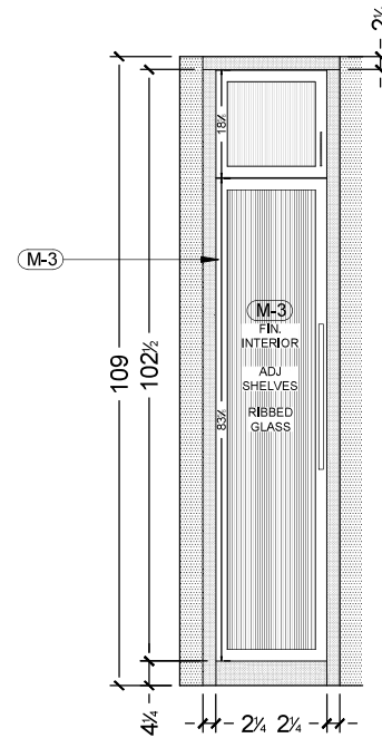
1 PRIVACY SCREEN SCALE: 1/2" = 1'0"
