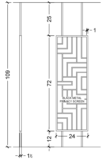
2 PRIVACY SCREEN SCALE: 1/2" = 1'0"
