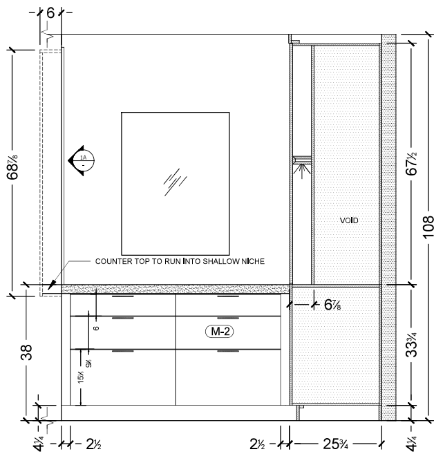
1 PRIMARY CLOSET SCALE: 1/2" = 1'0"
