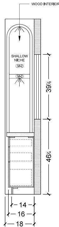
1A PRIMARY CLOSET SCALE: 1/2" = 1'0"
